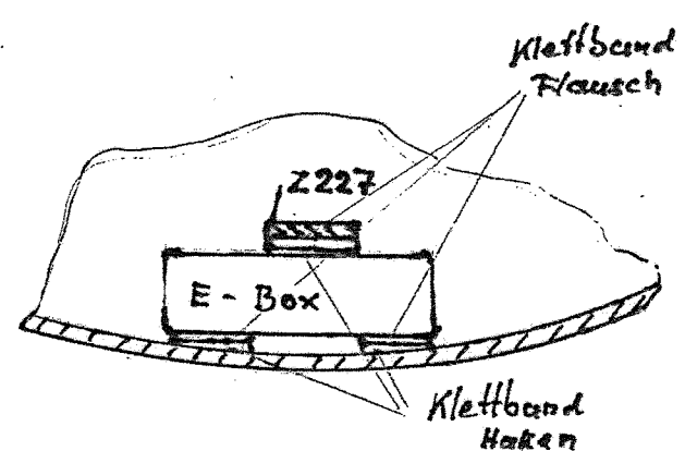
Schnitt X-X
